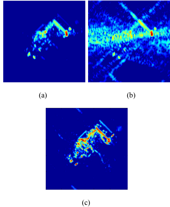
Şekil 2: (a) Faz hatasız durum için geleneksel görüntü (b) Faz hatalı durum için geleneksel görüntü (c) Faz hatalı durum için önerilen yöntemle oluşturulan görüntü.
